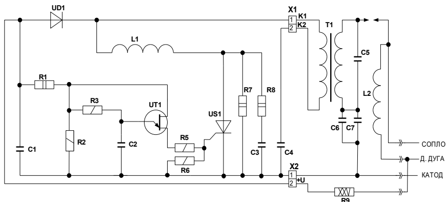
Рис.1 Схема электрическая принципиальная УВД-05
